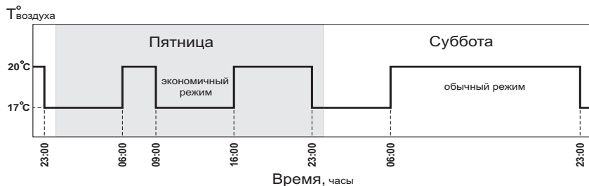
Рис. 7 График температуры воздуха в помещении для Режим 3.
