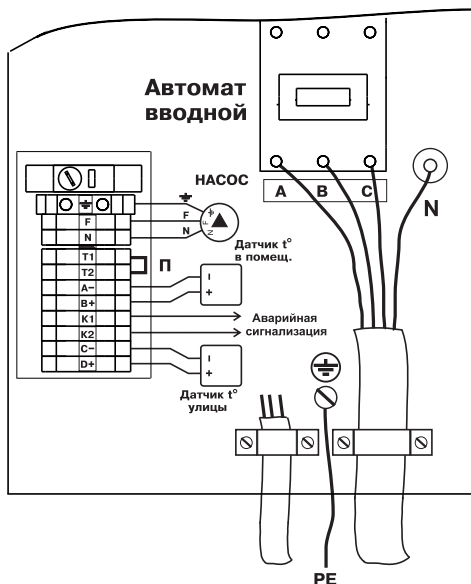
Рис. 3 Схема подключения электроводонагревателя
