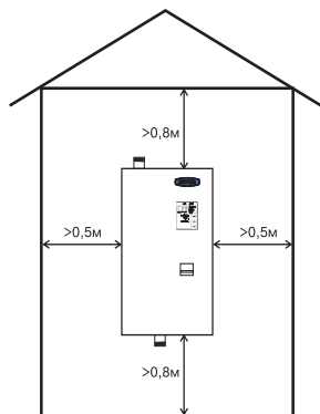
Рис. 4 Схема установки электроводонагревателя
